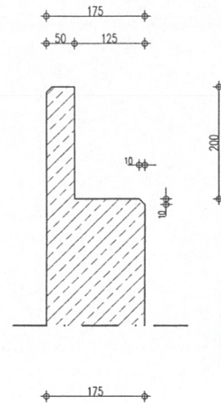
Abbildung 2: Wandkopf
