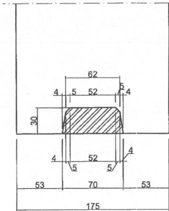
Abbildung 1: Wandfuß
