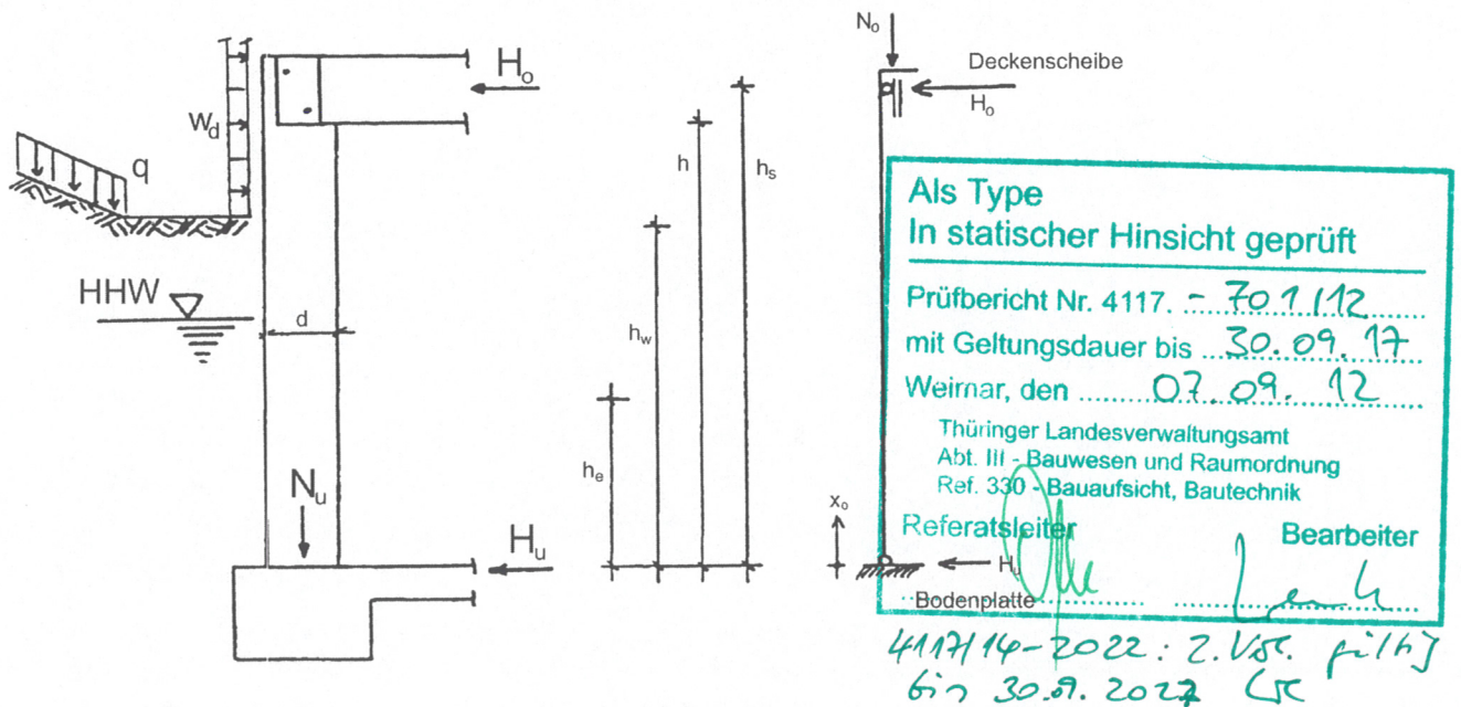
Abbildung 3: Prinzipskizze
